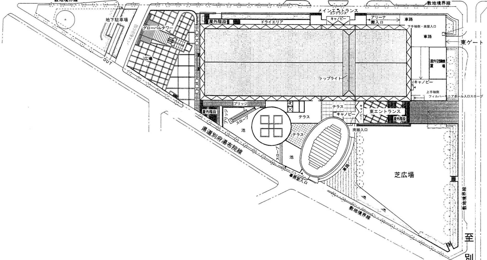
配置図
